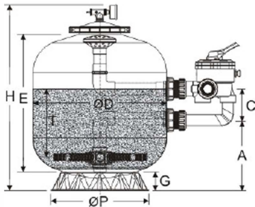
WL-ICG450~WL-ICG900
