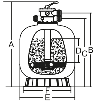
PNR-RFF700(B) - PNR-RCFF1400
