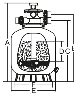
PNR-RFF350 - PNR-RFF700
