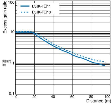
E3JK-T□11/T□13
