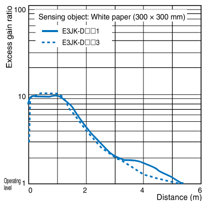
E3JK-D□□1/D□□3
