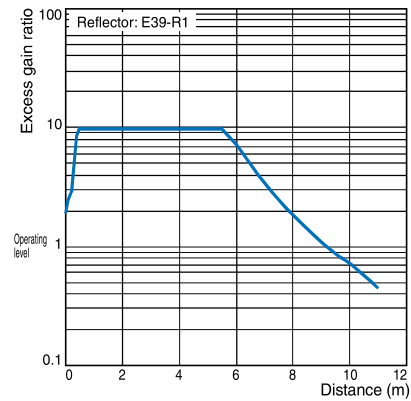
E3JK-R□□2+E39-R1
