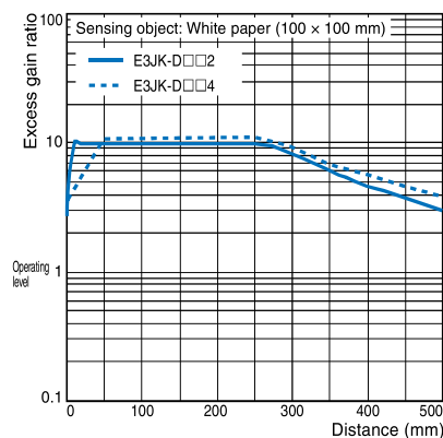
E3JK-D□□2/D□□4
