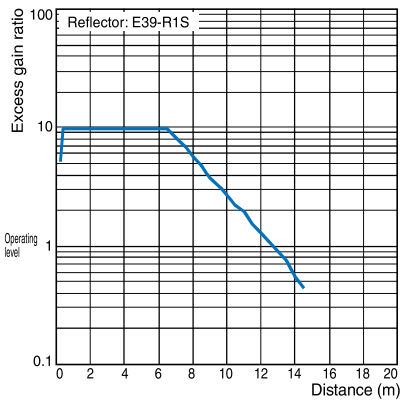
E3JK-R□□2+E39-R1S
