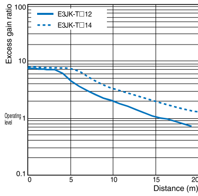
E3JK-T□12/T□14
