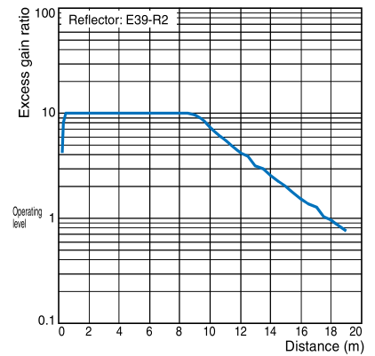
E3JK-R□□2+E39-R2
