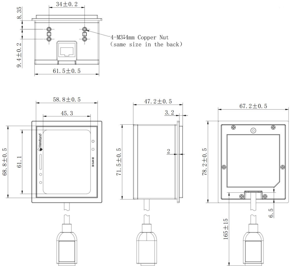
Dimensions: 78.7 (W) x 47.7 (D) x 67.7 (H) mm (max.) (without cable)
