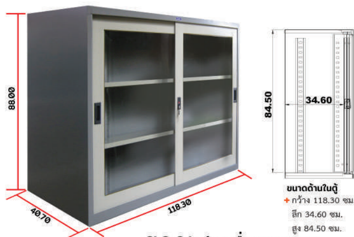
SLG-04 : ตู้บานเลื่อนกระจก 4 ฟุต W.118.5 x D.40.7 x H.88.0 CM. PRICE : 7,400.-
