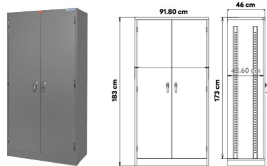
PK-211 ตู้เอกสาร 2 บานเปิด มีจับชนิดบิด (มอก.)
