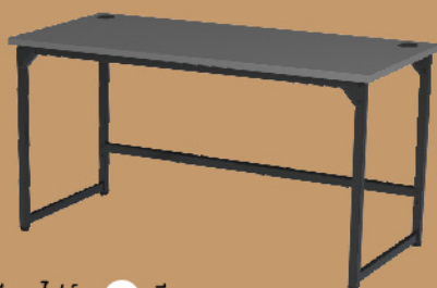
PDK-60150 โต๊ะทำงาน 150 cm W 150 x D 60 x H 75 cm PRICE 4,250.-
