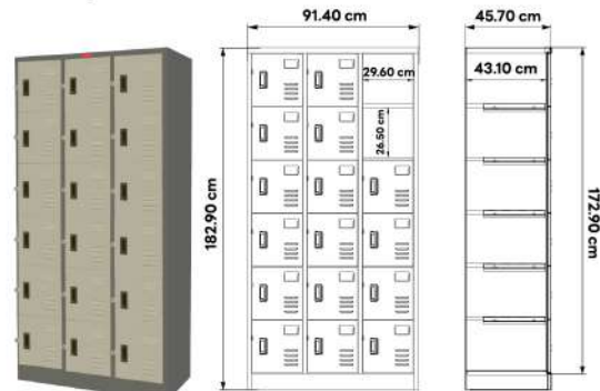
PK-018 ตู้ลิ้นชัก 18 ประดู่
