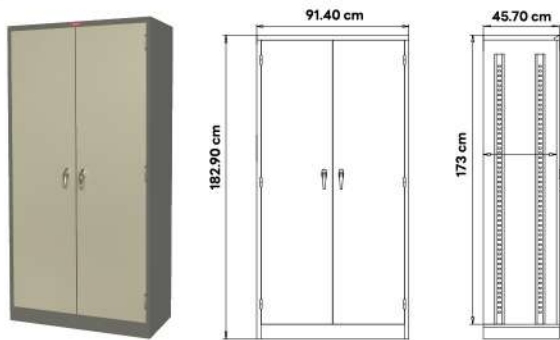
PK-100 ตู้เอกสาร 2 บานเปิด
