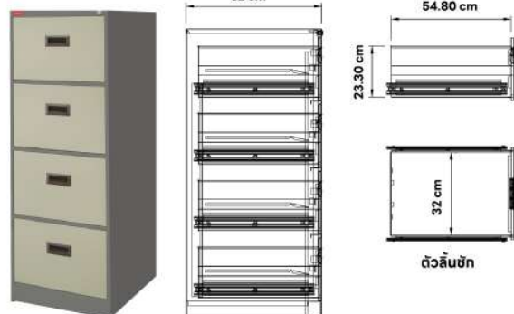
PC-104 ตู้เอกสาร 4 ลิ้นชัก ภายนอก W 46.1 x D 62 x H 132 cm ภายใน (ลิ้นชัก) W 32 x D 54.8 x H 23.3 cm PRICE 8,250.-
