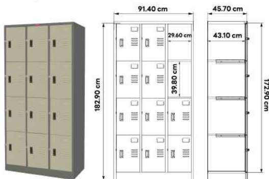
PK-012 ตู้ลิ้นชัก 12 ประดู่
