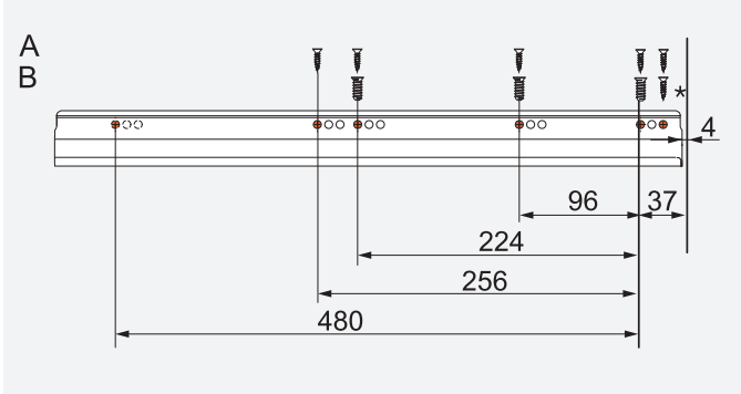
ตำแหน่งการยึดรางกับข้างตู้ - ความยาวรางลิ้นชัก 500 มม.
