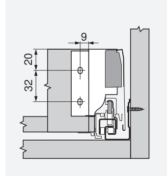
ขนาดการติดตั้ง - ด้านหลัง
