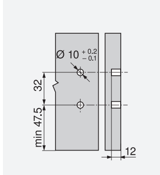
ระยะการเจาะ - หน้าบาน
