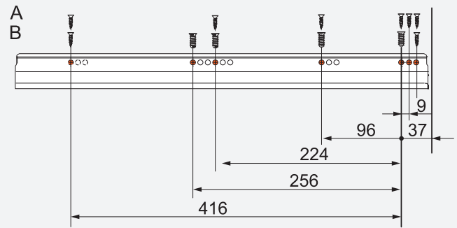
ราง - 576 ความยาว 500 มม.
