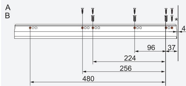
ตำแหน่งการยึดรางกับข้างตู้ - ความยาวรางลิ้นชัก 500 มม.
