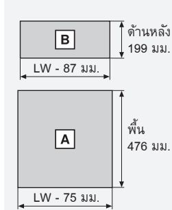
ขนาดตัดไม้ (แผ่นไม้ชิปบอร์ดหนา 16 มม.)
