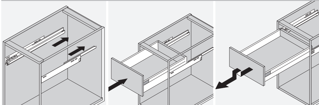
การใส่กล่องลิ้นชัก
