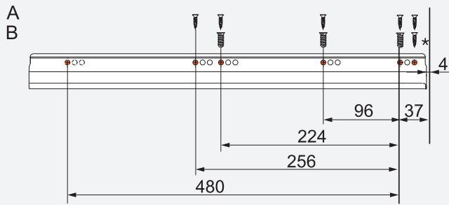
ราง - 578/579 ความยาว 500 มม.
