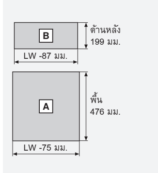
ขนาดตัดไม้ (แผ่นไม้ชนิดบอร์ดหนา 16 มม.)
