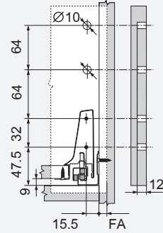
ขนาดการติดตั้ง - หน้าบาน
