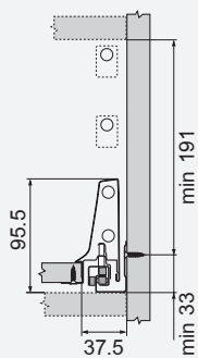
ขนาดที่ต้องการ
