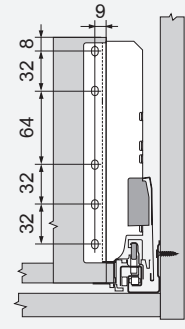
ขนาดการติดตั้ง - ด้านหลัง
