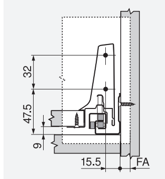
ขนาดการติดตั้ง - หน้าบาน
