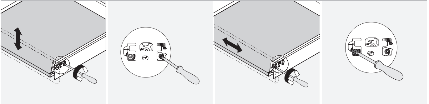
ปรับความสูง
