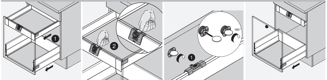
การล็อกกล่องลิ้นชัก
