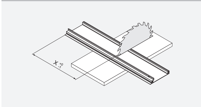
ขนาดการตัด - หน้าลิ้นชัก
