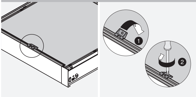
แนะนำให้ใช้เมื่อลิ้นชักกว้างเกิน 600 มม.
