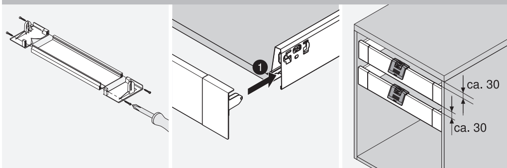
การประกอบ
