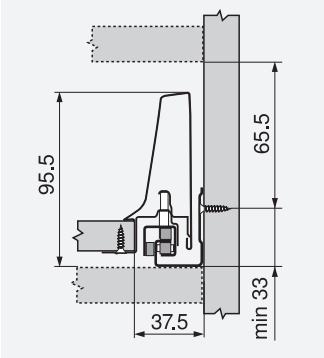
ขนาดที่ต้องการ
