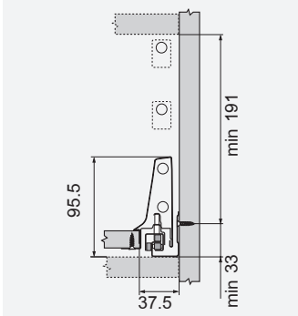
ขนาดที่ต้องการ
