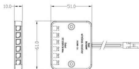
LEDSS-6050-5A
