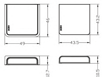
LEDSS-4946DC
