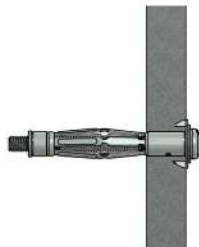
สอดพุกลงในรูเจาะ
