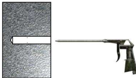
เป่าลมที่รูเจาะ
