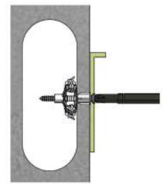
ขันสกรูจนงานติดแน่น
