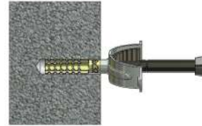
ขันยึดชิ้นงานให้แน่น
