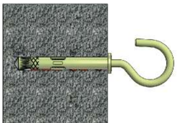
สอดพุกลงในรูเจาะ
