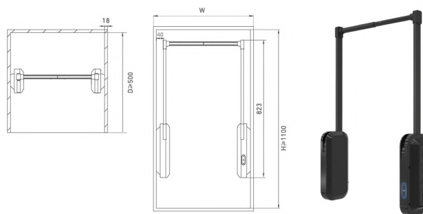
ราวแขวนผ้าปรับขึ้น-ลงอัตโนมัติ ELECTRIC PULL-DOWN HANGER
