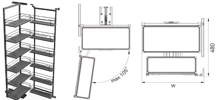
ชุดตะแกรงทรงสูง 6 ชั้น รุ่นเปิด-ปิดประตูลูก LATERAL PANTRY BASKETS
