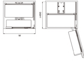
ชุดตะแกรงทรงสูง 6 ชั้น ร่มเปิด-ปิดประตู LATERAL PANTRY BASKETS
