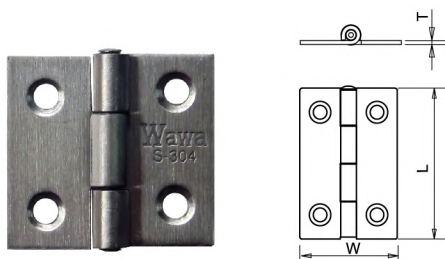
บานพับสแตนเลส STAINLESS STEEL HINGE (IM)
