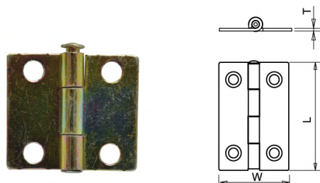
บานพับเหล็ก รุ่นหนา STEEL HINGE (PA)
