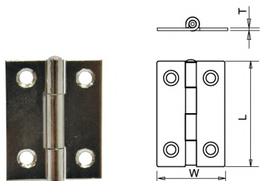
บานพับเหล็ก รุ่นบาง STEEL HINGE (PA)
