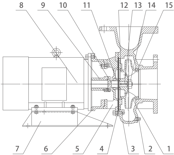
HWPDP结构简图
