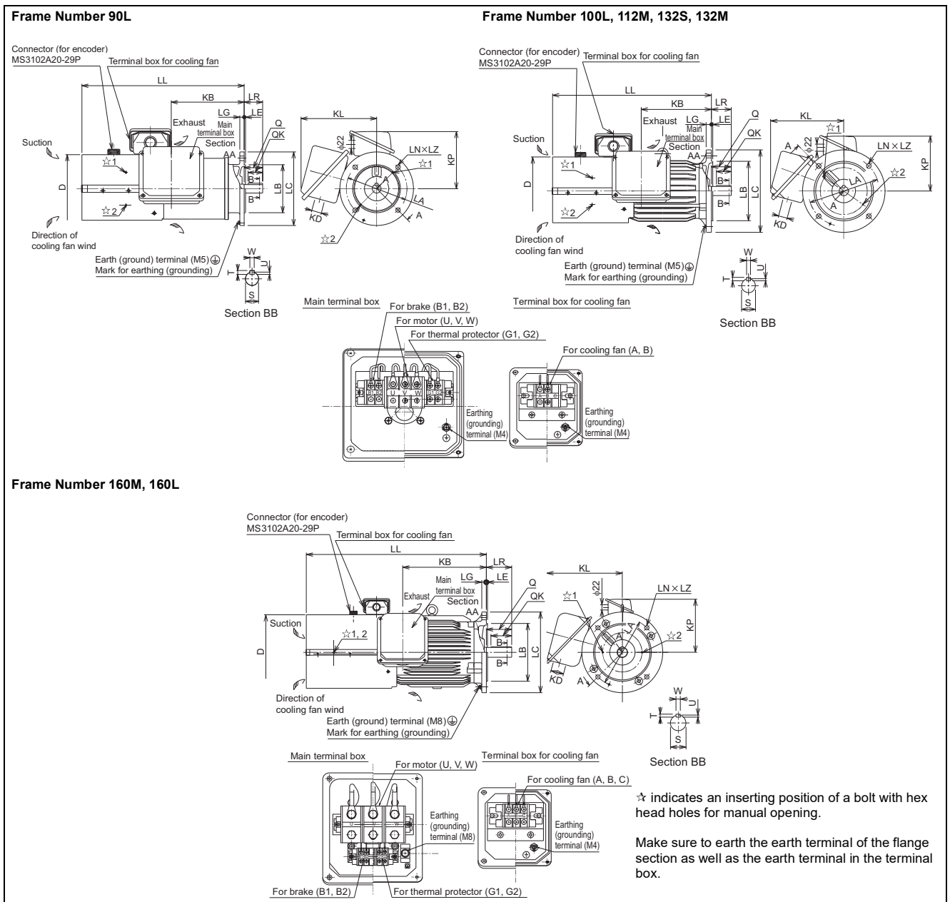
Dimensions table
