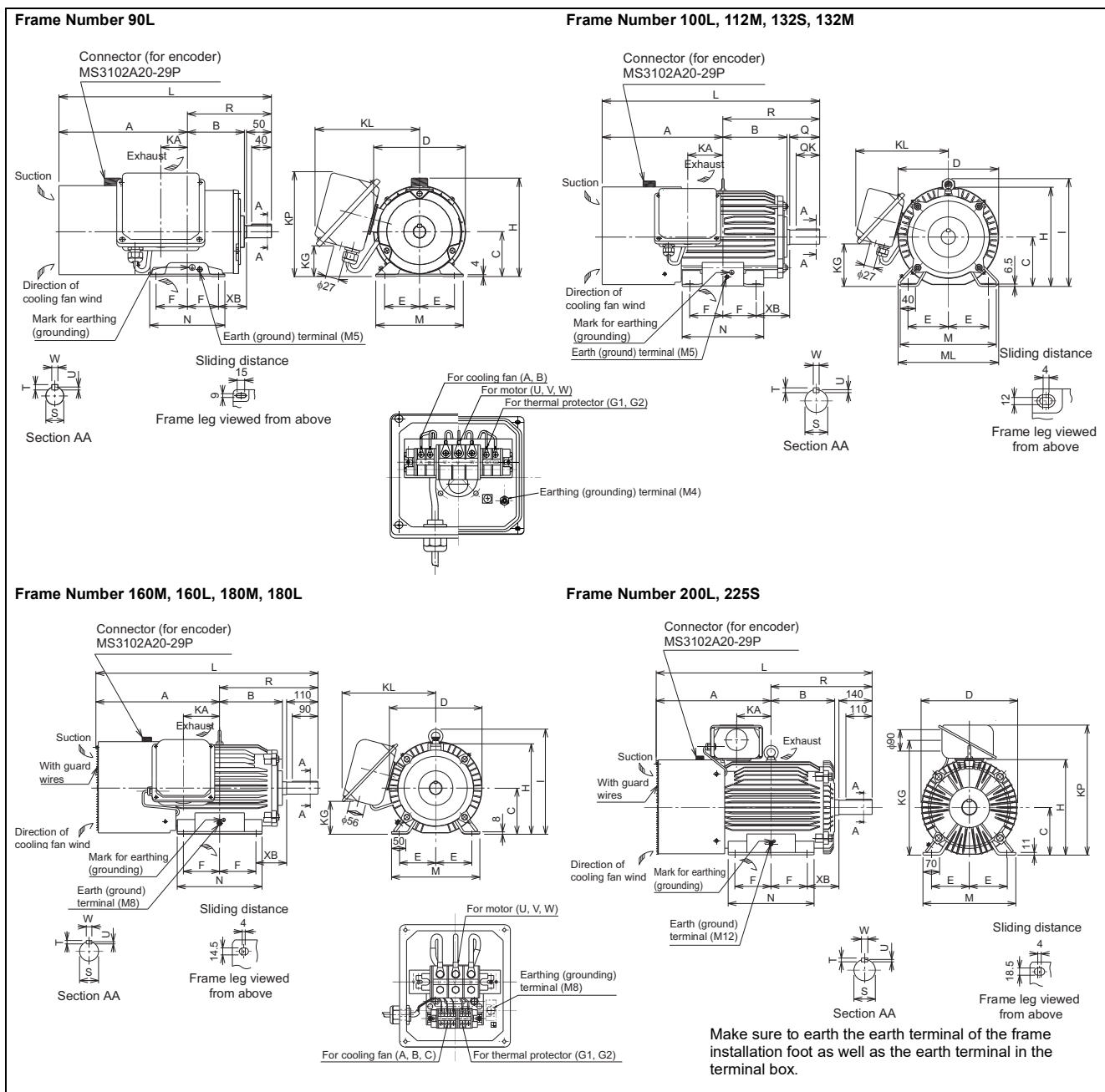
Dimensions table
