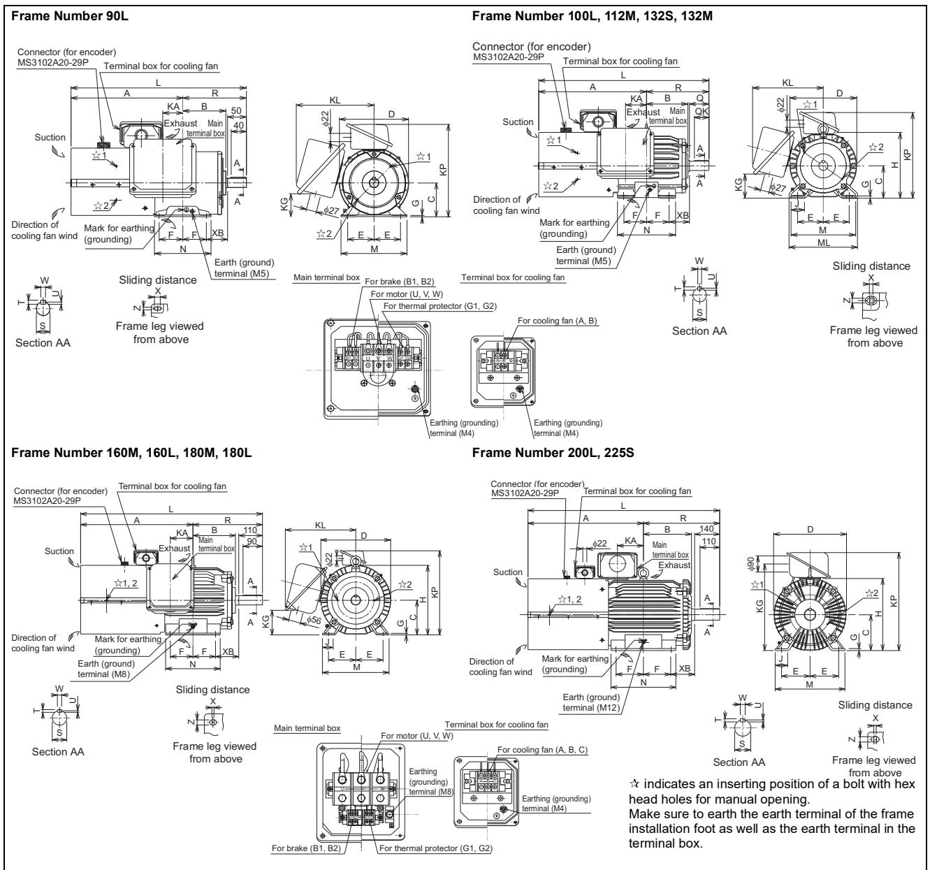
Dimensions table
