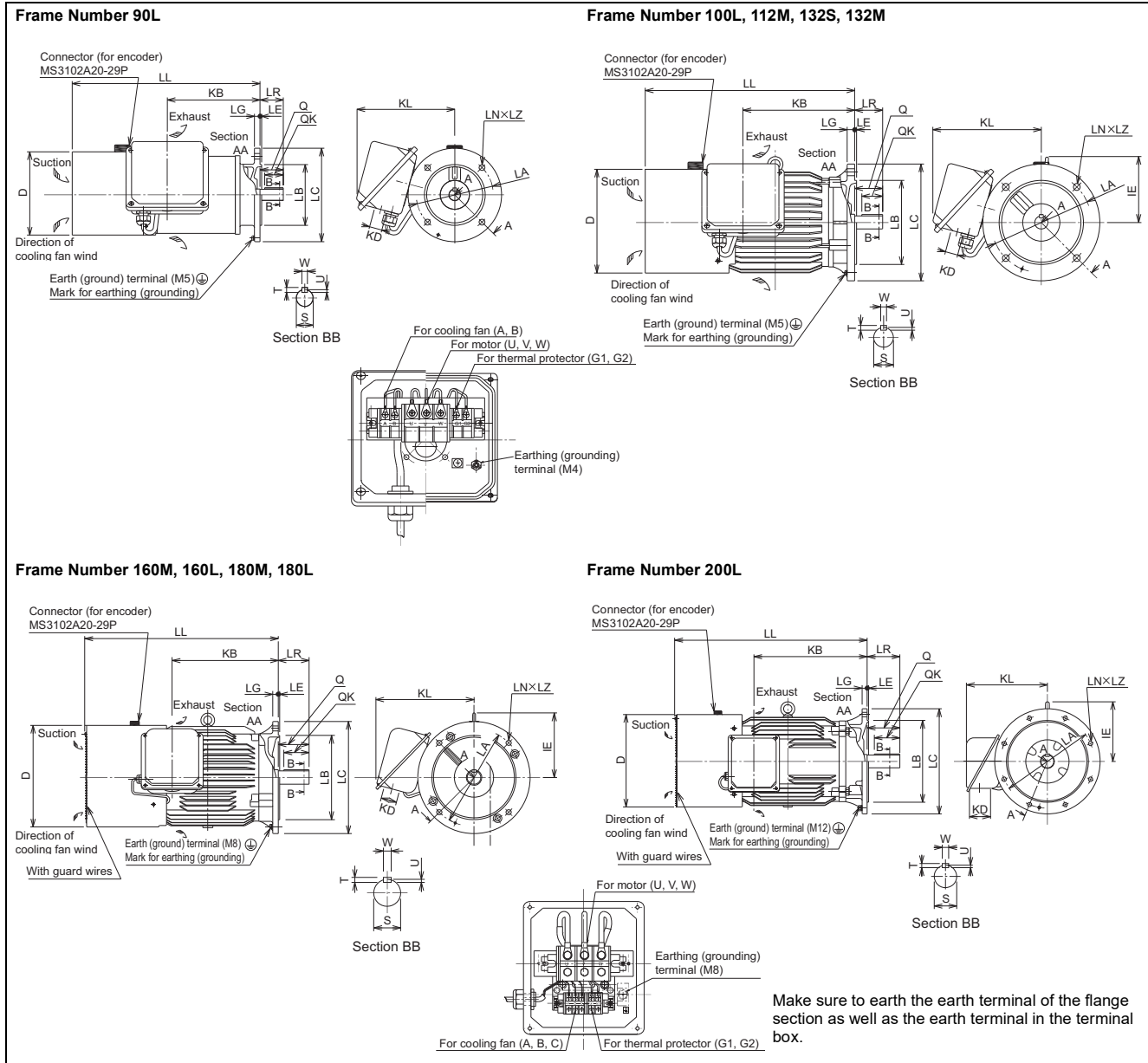
Dimensions table
