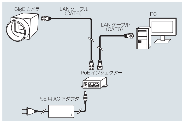
POE電源接続図
